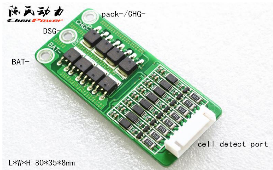
CPR-EP600-C8 磷酸铁锂电产品实物图
